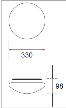
PL35 - 22W
