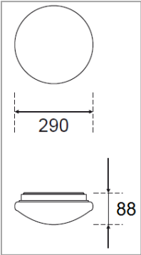
PL29 - 12W
